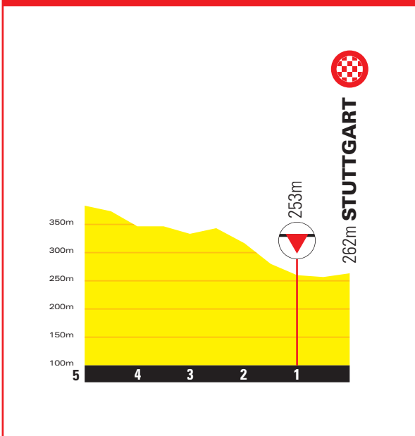
HÖHENPROFIL FINALE LAST 5KM PROFILE
